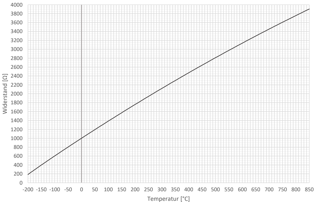
Kennlinie Pt1000
