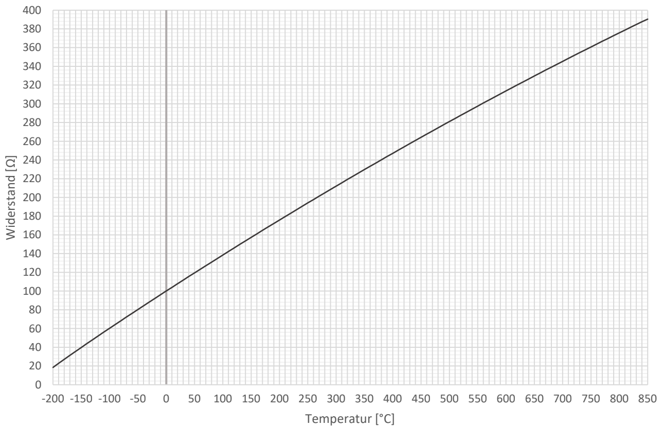
Kennlinie Pt100
