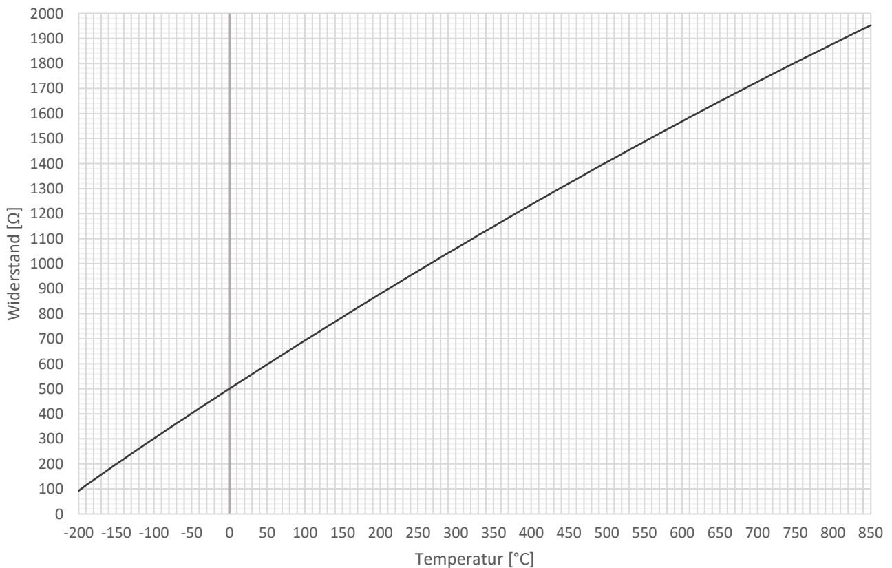
Kennlinie Pt500
