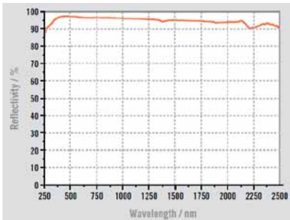
Reflexionseigenschaften des QRC Nanoreflectors
