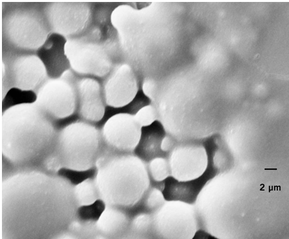
QRC Material mit Mikro- und Nanostruktur unter dem Raster-Elektronenmikroskop
